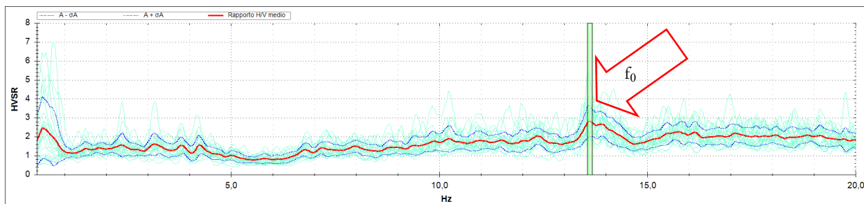
Figura 5 - Snapshot Curve HVSR (su scala lineare). Si indica il picco fondamentale f_0 (con A_0 \geq 2.8 ).
