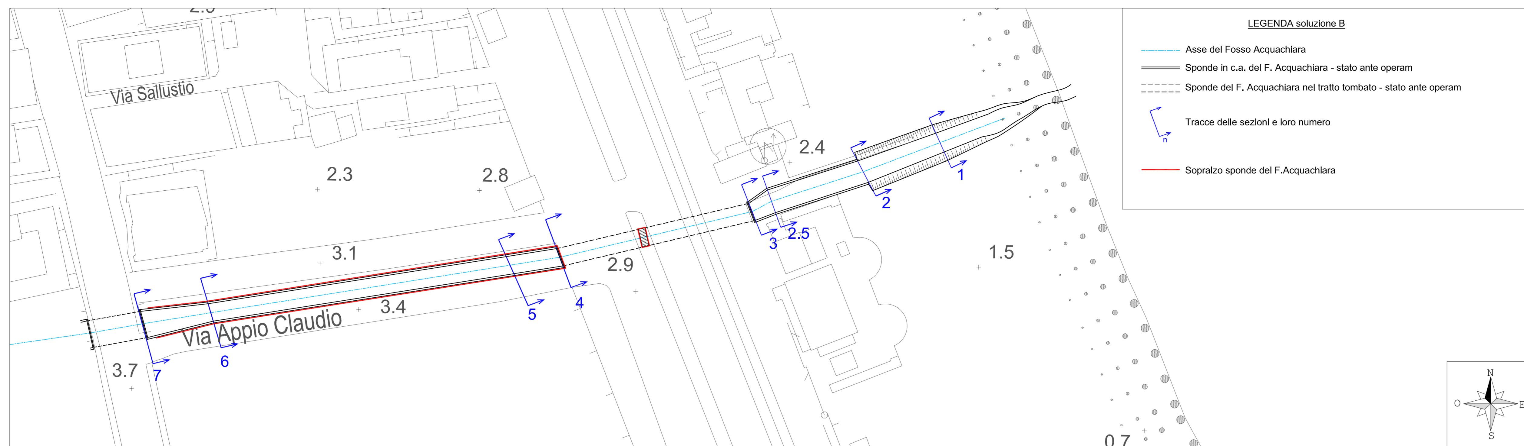
Planimetria - scala 1:500
