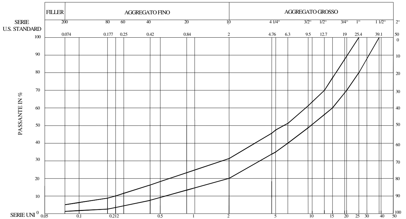
Limiti e corrispondente fuso granulometrico per la MISCELA SECCA DEGLI INERTI
